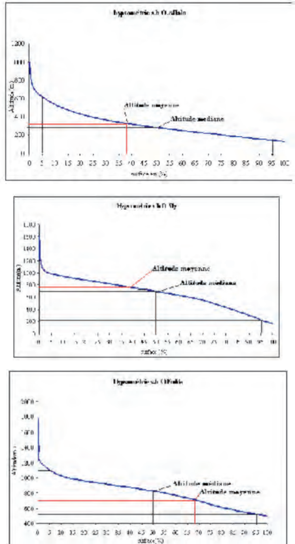
Fig. 3 - courbes hypsométriques O.Allala O.Fodda. O.Sly
