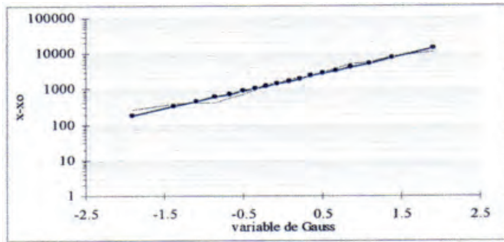
Fig. 11 - Distribution selon la loi log-normale de l'érosion spécifique (Oued Allala)
