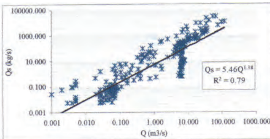
Fig. 6 - Relation débit liquide-débit solide station L.O.Farés.(o.Sly)
