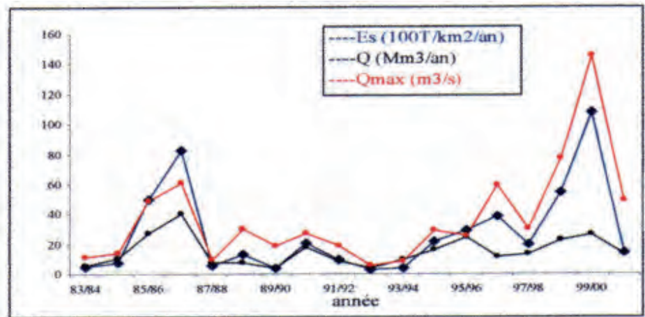
Fig. 12 - Variation de l'érosion spécifique avec l'apport annuel et le débit journalier max.
