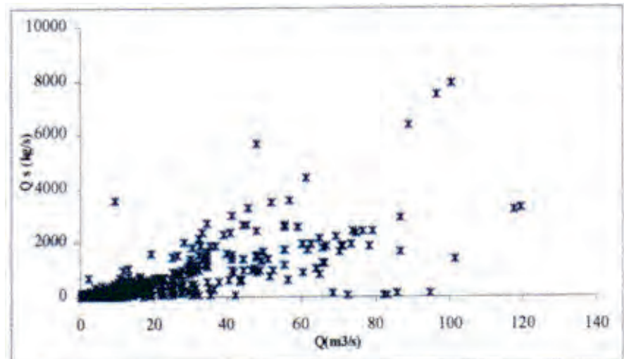
Fig. 9 - Relation débit solide -débit liquide station O.Fodda (1983/2001)
