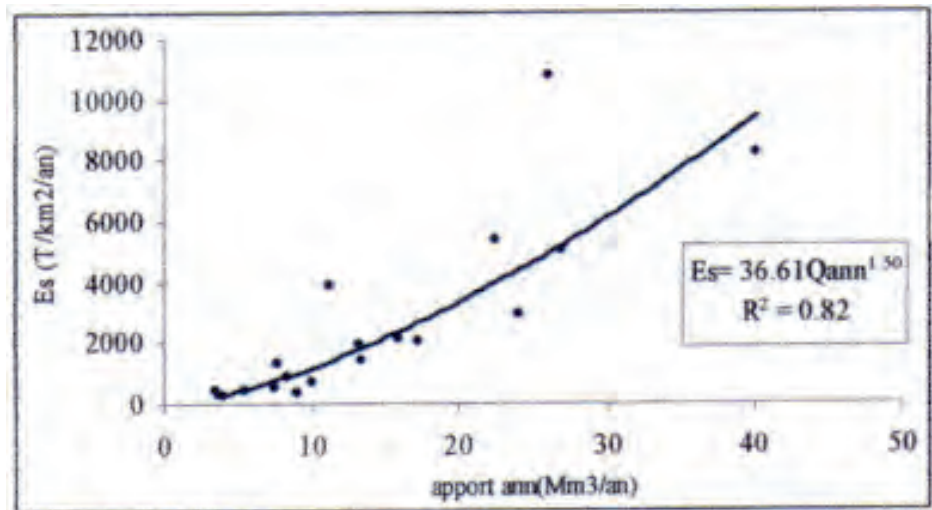
Fig. 13 - Relation puissance entre l'érosion spécifique et l'apport annuel.
