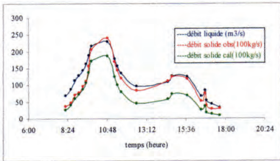
Fig. 10 - Débit solide observé et calculé avec le débit liquide lors d'une crue à la station Sidi Akkacha.
