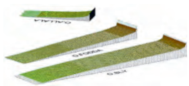
Fig. 2 - Rectangle equivalent de O. Allala. O. Fodda. O. Sly
