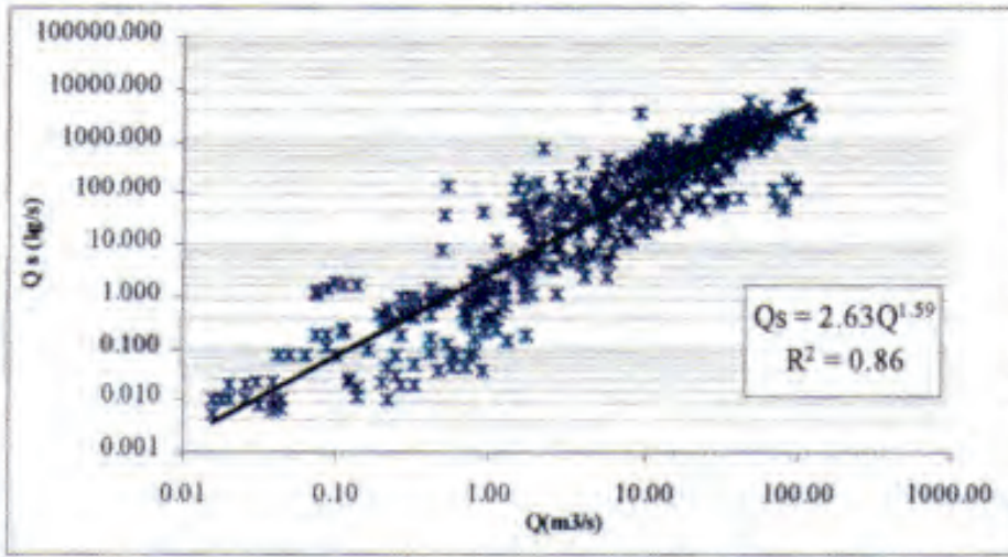
Fig. 4 - Relation débit liquide-débit solide station O.Fodda.
